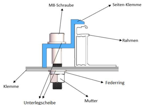
Abb. 9 Installation schematische Darstellung der Randklemme
