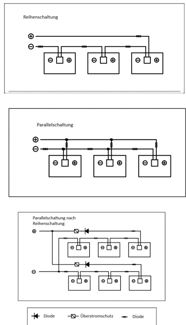
Abb. 11 Schaltbild der elektrischen Anschlüsse
