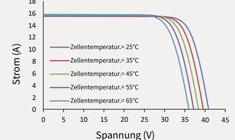
Strom-Spannung (510 W)
