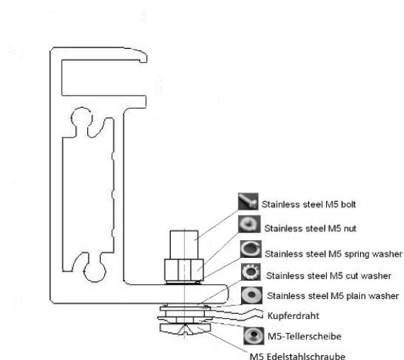
Abb. 14 Erdung des Aluminiumrahmens mit Kupferdraht
